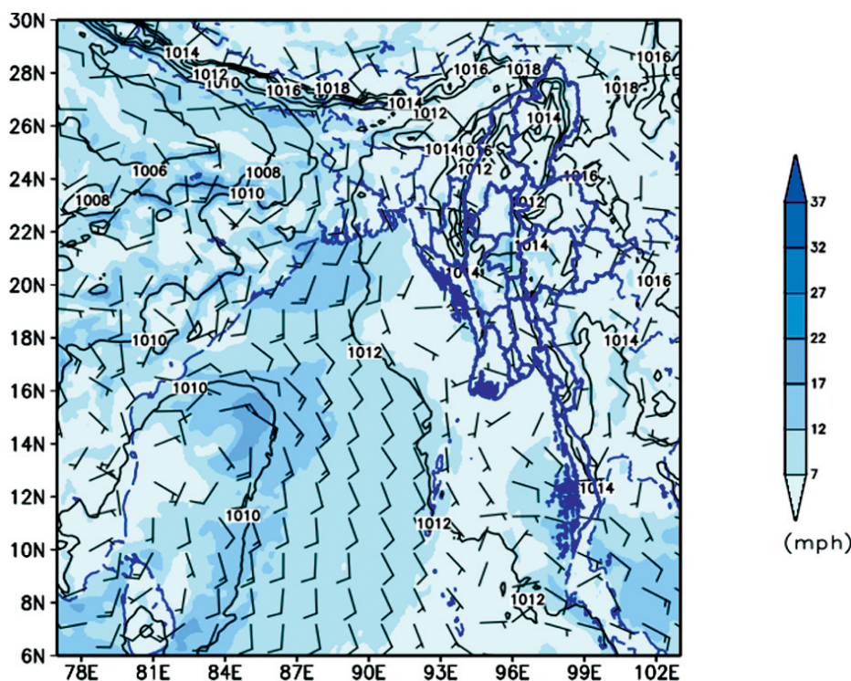
မိုးလေဝသနှင့် ဇလဗေဒညွှန်ကြားမှုဦးစီးဌာန၊ WRF မော်ဒယ်၏ ၃၁-၃-၂၀၂၅ ရက်နေ့ မြန်မာစံတော်ချိန် ၀၆:၃၀ နာရီအချိန်ကို အခြေခံတွက်ထုတ်ထားသည့် ၈-၄-၂၀၂၅ ရက်နေ့ မြေပြင် လေတိုက်ခတ်မှုအခြေအနေနှင့် လေထုဖိအားပြပုံ။
