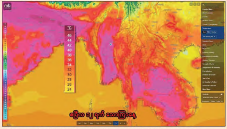
ဧပြီလ ၁၂ ရက်တွင် ဖြစ်ပေါ်လာနိုင်သည့် နေအပူချိန်ပြ ခန့်မှန်းရုပ်ပုံကားချပ်။
