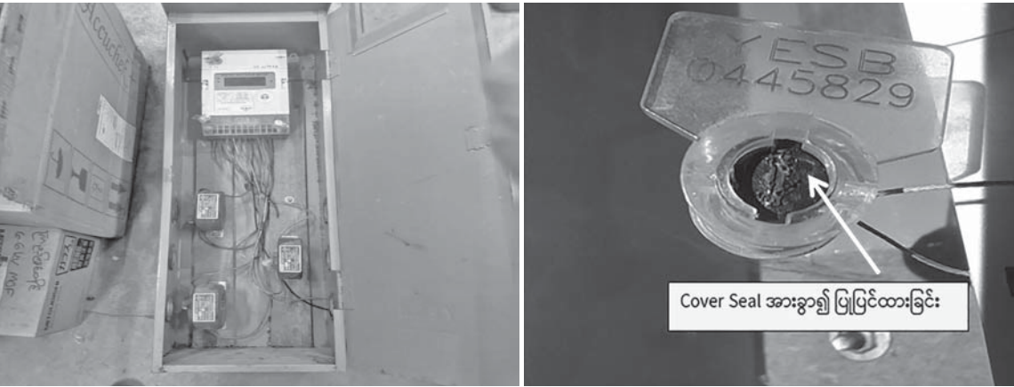
မှော်ဘီမြို့နယ် ဝါးနက်ချောင်းကျေးရွာရှိ မိတာအမည်ပေါက် ဦးစန်းဦး၏ ကော်စေလုပ်ငန်းတွင် အသုံးပြုထားသော Transformer နှင့်တွဲဖက်တပ်ဆင်ထားသည့် Digital Meter ၏ Cover Seal ပြုပြင်ထားသည့်မှတ်တမ်းဓာတ်ပုံများကို တွေ့ရစဉ်။
