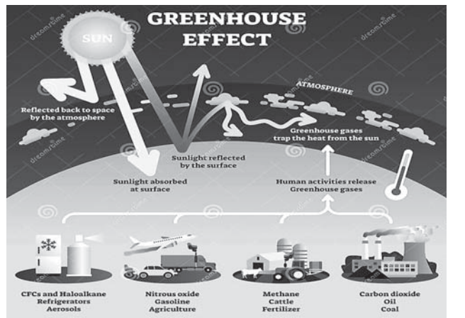
ကမ္ဘာကြီးပူနွေးမှုဖြစ်စဉ် Greenhouse Effect
