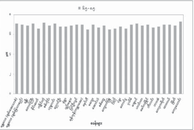
၂၀၂၄ ခုနှစ်၊ အောက်တိုဘာလအတွင်း ရွာသွန်းခဲ့သော မိုးရေမူနာများ၏ pH တန်ဖိုးများ
