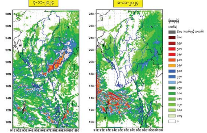
မိုးလေဝသနှင့်ဓလေပေဒည့်ကြားမှုဦးစီးဌာန၊ WRF မော်ဒယ်၏ ၆-၁၁-၂၀၂၄ ရက်နေ့ မြန်မာစတင်ချိန် (၀၆:၃၀)နာရီအချိန်ကို အခြေခံတွက်ထုတ်ထားသည့် ၇-၁၁-၂၀၂၄ မှ ၈-၁၁-၂၀၂၄ ရက်နေ့အထိ မိုးရွာသွန်းမှုခန့်မှန်းချက်ပြပုံ
